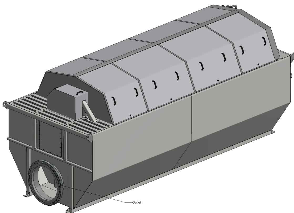
Figur 3.2 HDF12/16/20/24, filter med tank.
