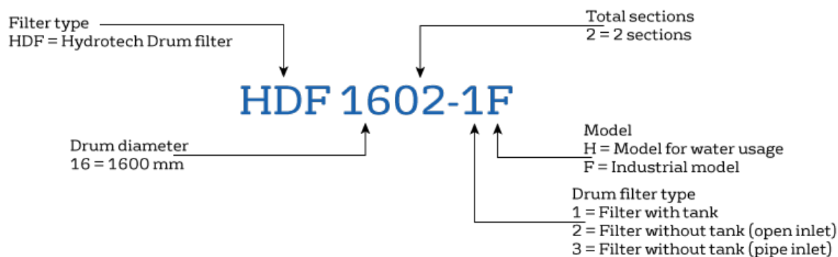
Figur 3.4 Definition av filtermodell.
