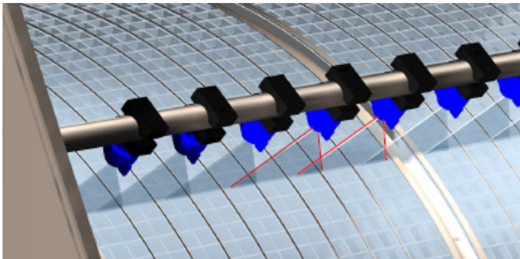
Figur 8.1 Korrekt spridningsbild för spolvatten.
