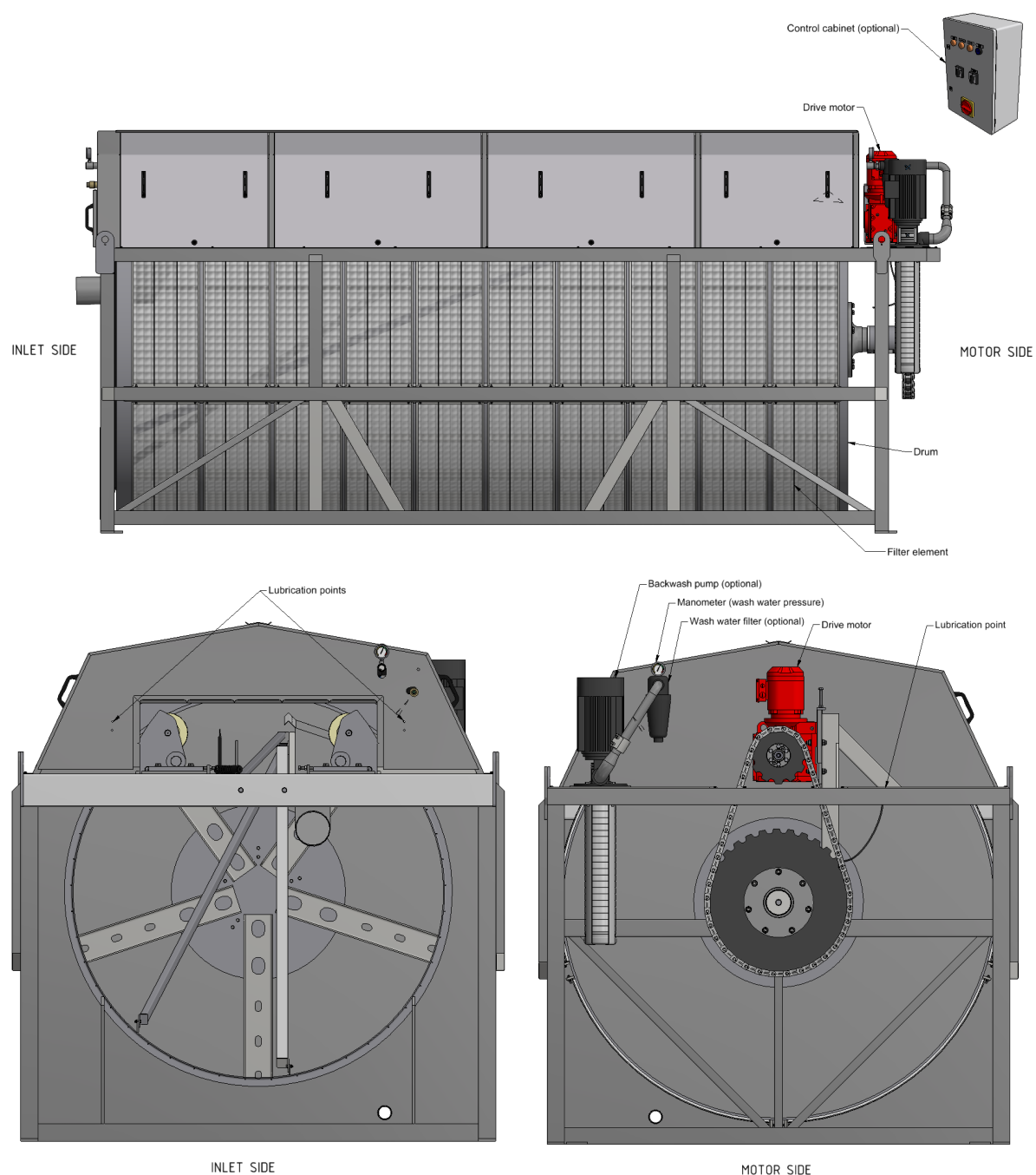
Figur 3.1 HDF12/16/20/24-seriens delar, filter med ställning.
