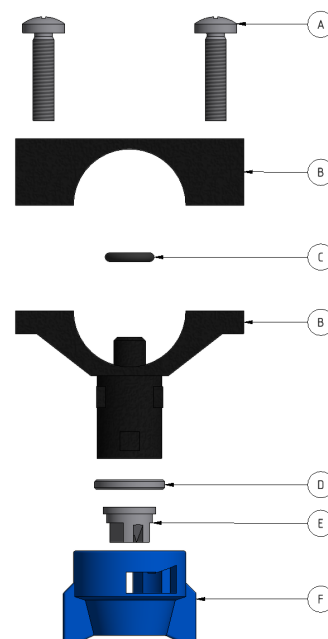
Figur 8.2 Dysdetaljer:
