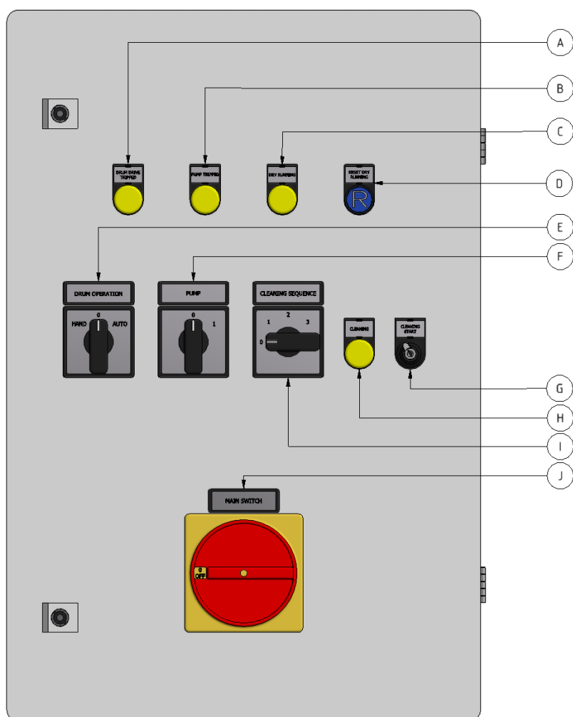
Figur 6.1 Hydrotech kontrollskåp typ PFC (tillval).
