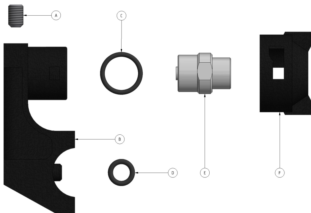
Figur 8.3 Dysdetaljer, självrengörande dysa (Yucheon).
