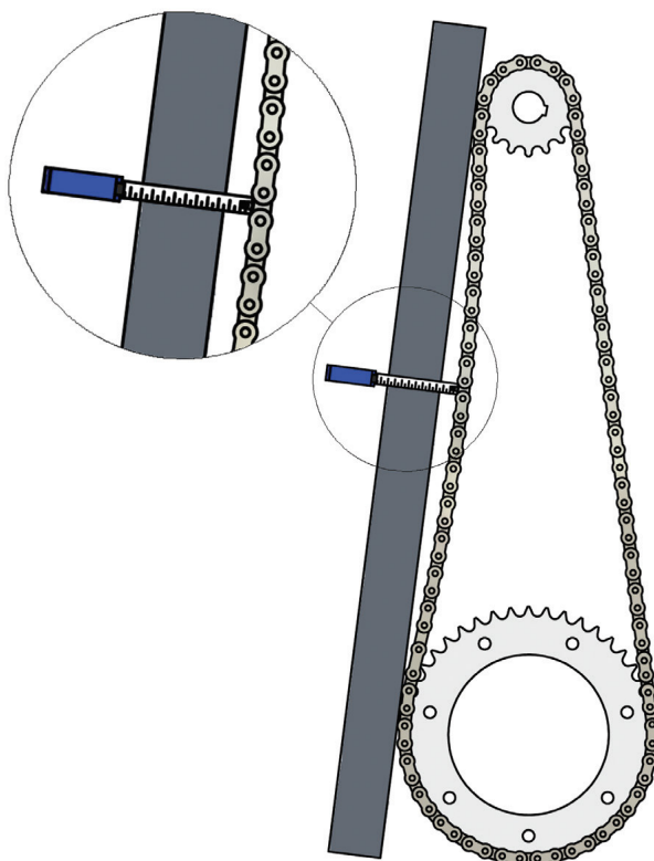
Figur 8.8 Kontroll av drivkedjans sträckning.
