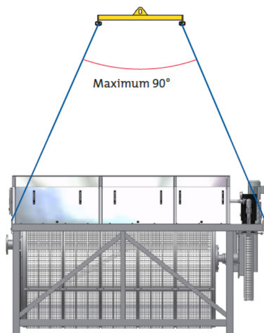
Figur 4.1 Lyftpunkter för filter utan tank (typ 2/3).
