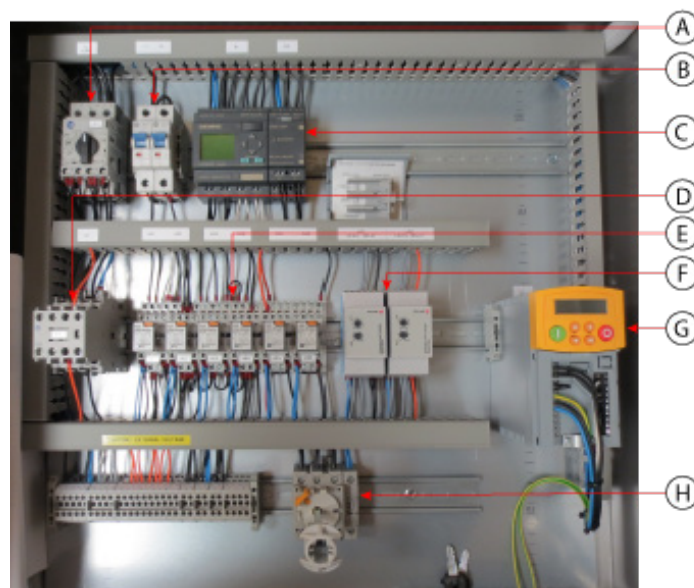
Figur 6.2 Hydretech standardkontrollskåp, typ PFC (tillval) (Kontrollskåpets konstruktion är i allmänhet anpassad till respektive applikation).
