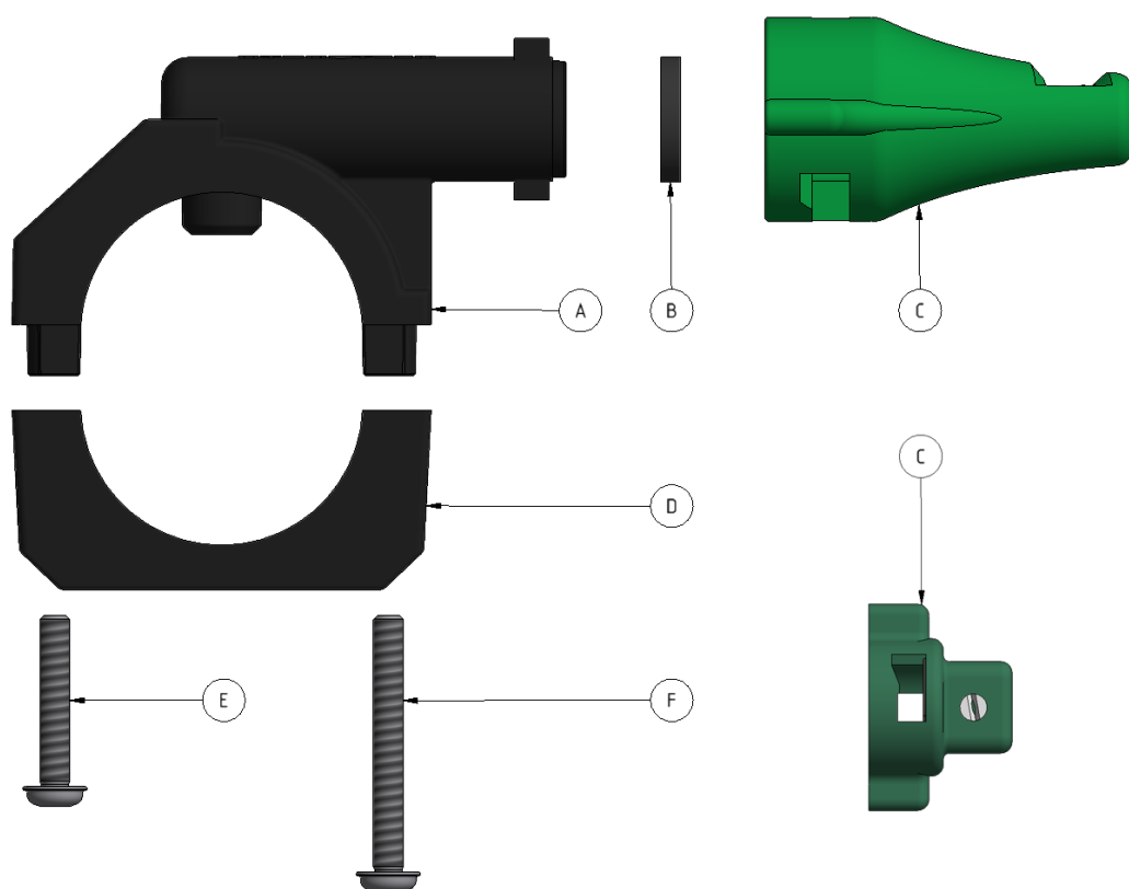
Figur 8.3.1 Lechler dyskomponenter. A. Övre dysfäste B. Gummitätning C. Överst: Dysmutter, självrengörande (tillval) Underst: Standard dysmutter D. Undre dysfäste E. 20 mm skruv F. 30 mm skruv
