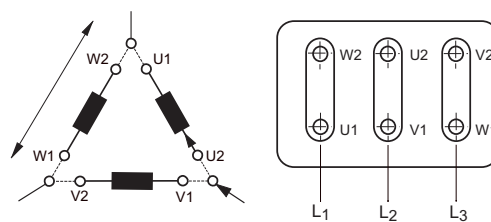
Fig. 14 D-koppling
