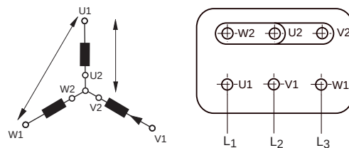
Fig. 15 Y-koppling
