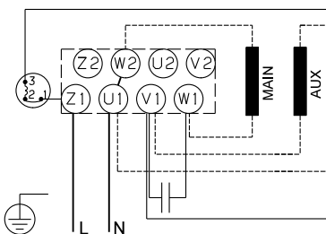
Fig. 17 Anslutning, "hög spänning", 0,37 - 0,75 kW
